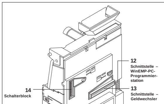
Abb. 1c: Rückseite des Münzprüfers
