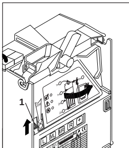
Abb. 10: Laufbahnträger des Münzprüfers aufklappen u. schließen
