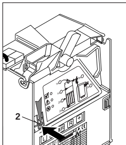
Abb. 10: Laufbahnträger des Münzprüfers aufklappen u. schließen
