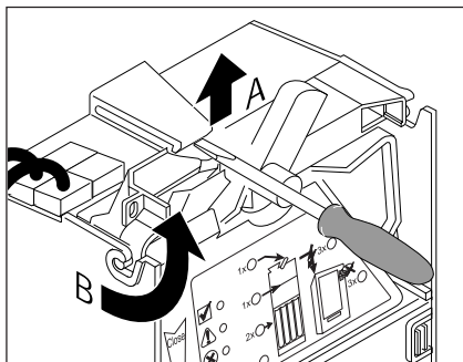
Abb. 1b: Münzprüfer ausbauen
