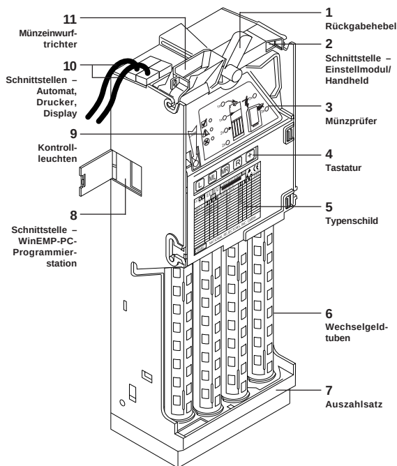
Abb. 1a: Aufbau
