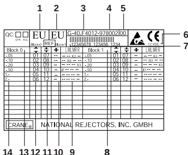
Abb. 2: Typenschild des Geldwechslers
